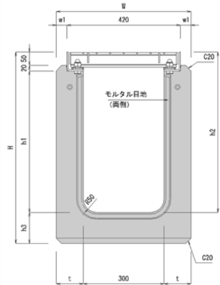
越流抑制グレーチング
